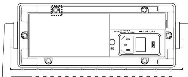
Рисунок 2. Схема пломбировки вольтметров (задняя панель).
